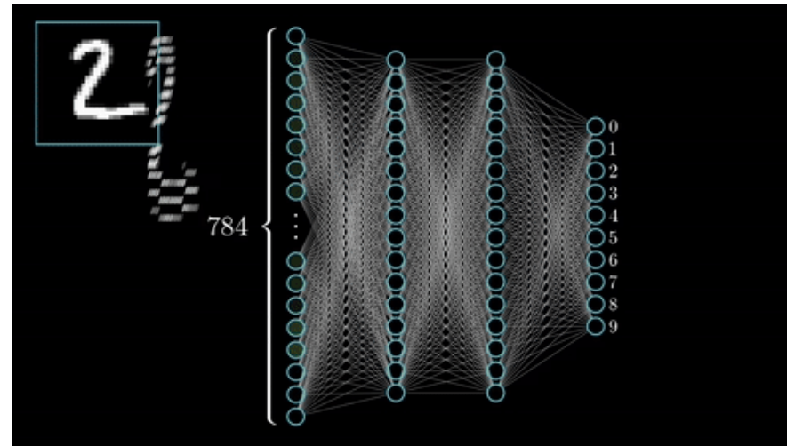
Fig.13 - Aplanar una imagen hace que perdamos su información espacial. Fuente: Suraj Yadav (Medium) .
