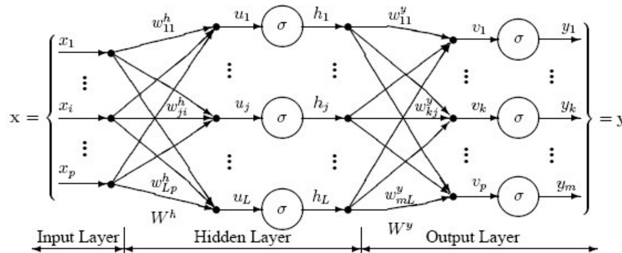
Fig.4 - Esquema de un perceptrón multicapa. Fuente: AllElephant .
