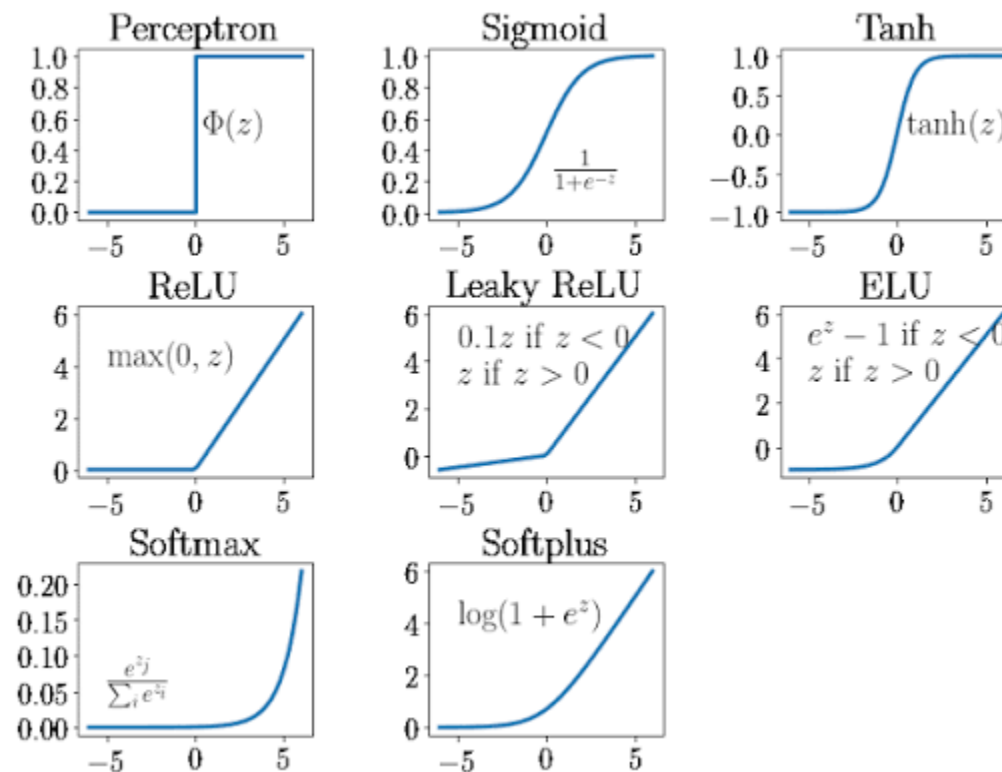
Fig.5 - Algunas funciones de activación. Fuente: Johnson et al. 2020 .
