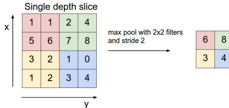
Fig.18 - Ejemplo de operación de max pooling . Autor: GeeksForGeeks .
