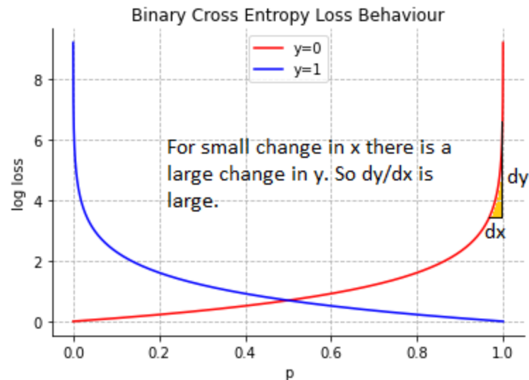
Fig.6 - Entropía cruzada (clasificación). Fuente: Datamonje .
